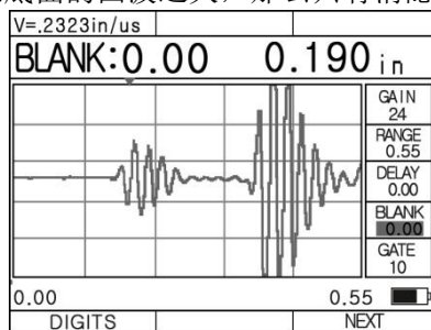
图3.9 消隐前波形
